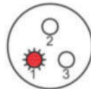
N + 1 live wire 2,3 shortage
